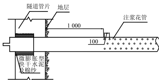
图2 注浆花管下放示意图(单位:mm)
