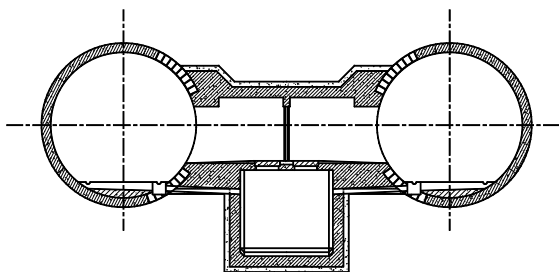
图1 联络通道结构示意图
