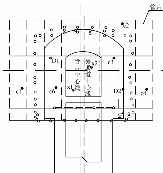
图 4 测点布置图
